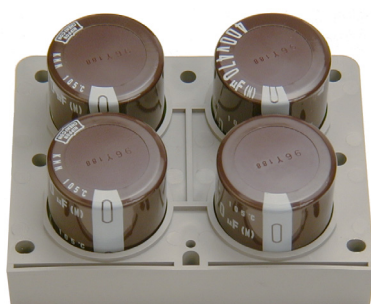
Moduł kondensatorów DC (Patrz rozdział 6- serwis)
