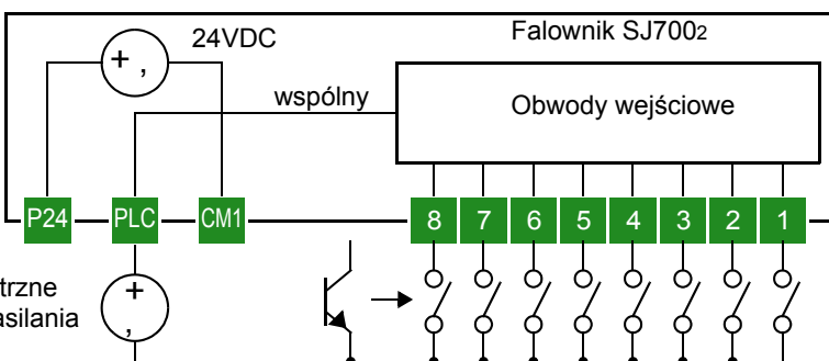
Wspólny minus, zasilacz zewnętrzny
