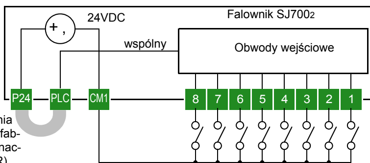
Wspólny minus, zasilacz wewnętrzny
