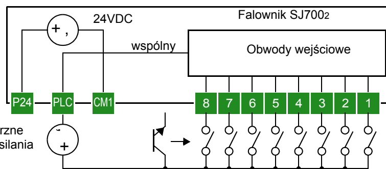
Wspólny plus, zasilacz zewnętrzny
