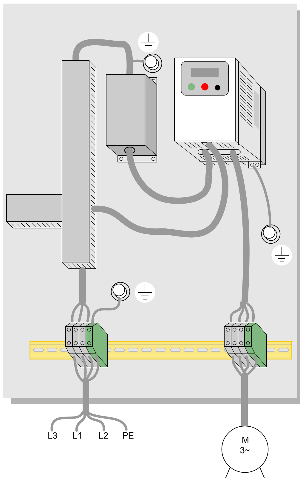
Falownik SJ200 z filtrem montowanym obok
