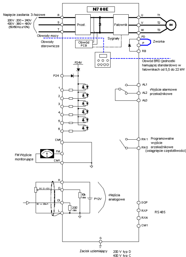
Fig 3-2 Diagram połączenia przy sterowaniu z panela
