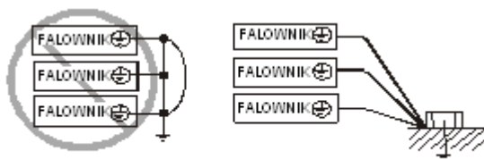
Rys. 2- 4 Uziemienie (G)
