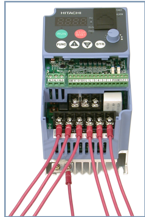
Podłączenie falownika L200-004NFU
